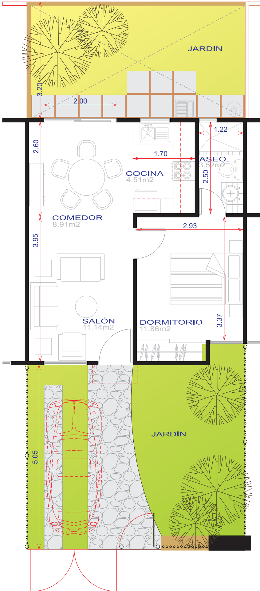
PLANTA TIPO
